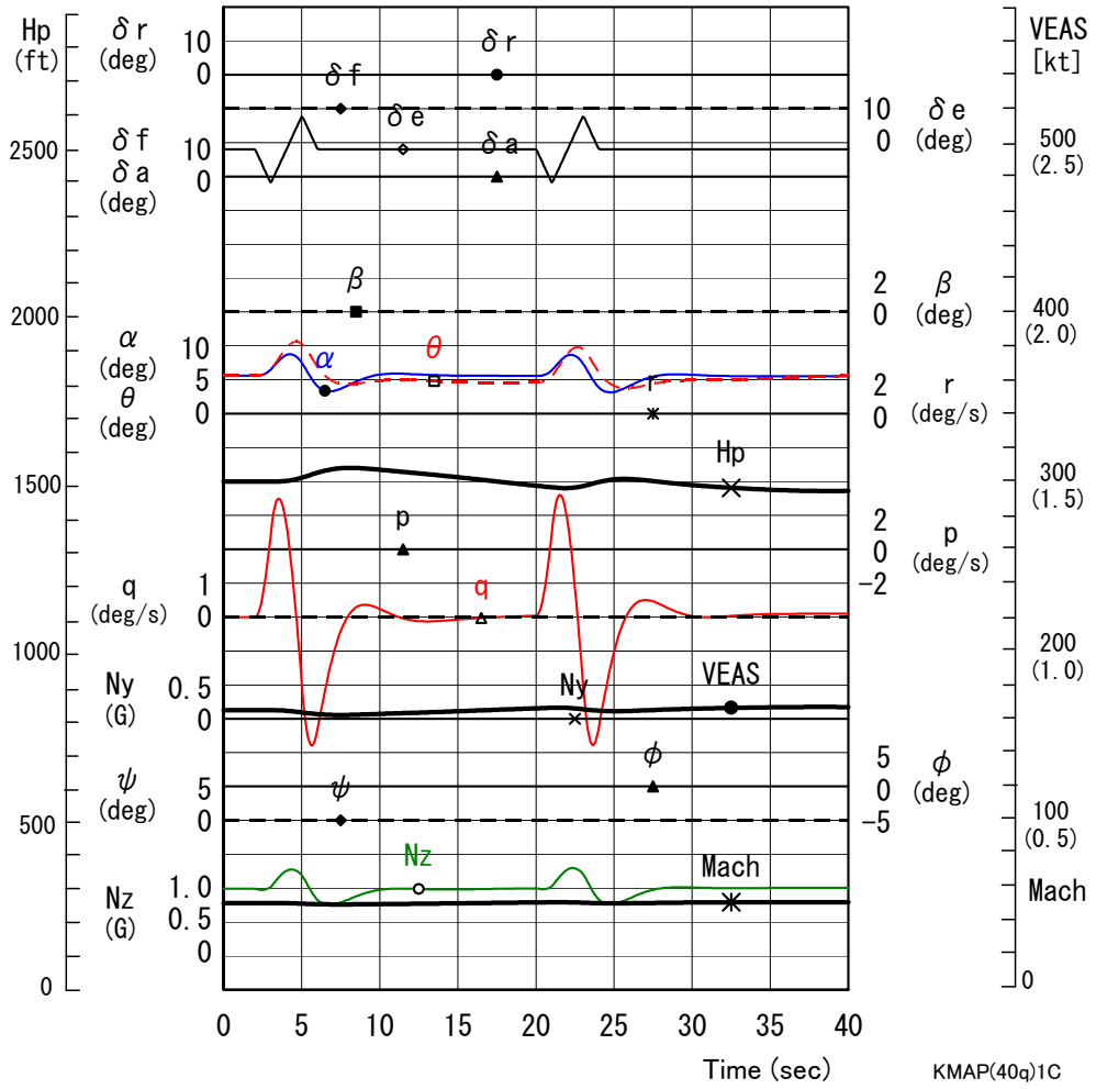
(W381.DAT) 1,500FT,165KT 1G (PA),機体固有,短周期モード例
